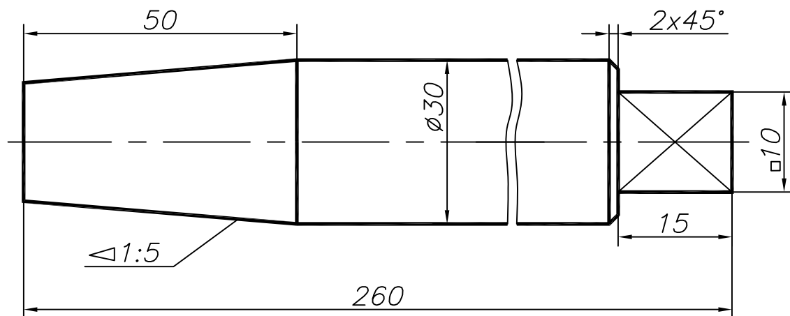
Цапфа
