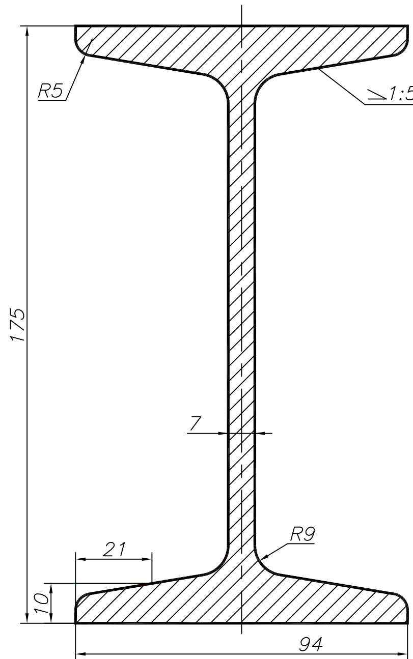
Двутавр 20а
